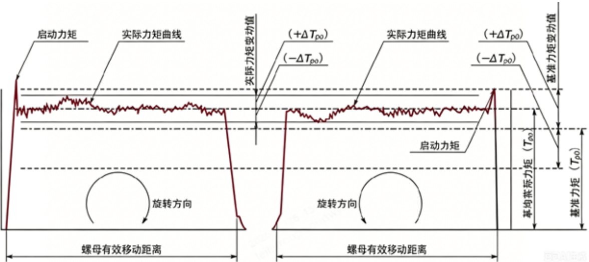
扭矩测量示例
