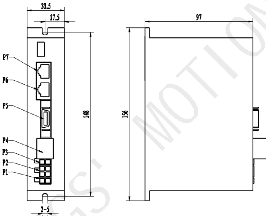
外形尺寸 (mm)
