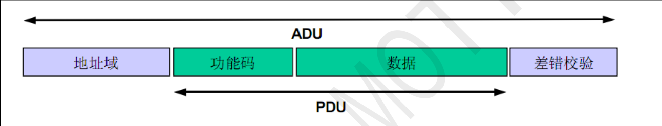
通用 MODBUS 帧
