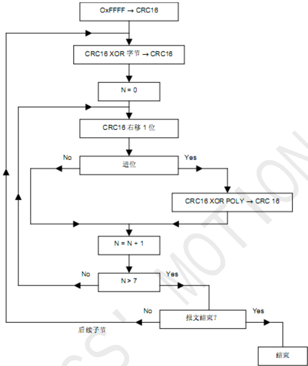
CRC 16 计算算法
