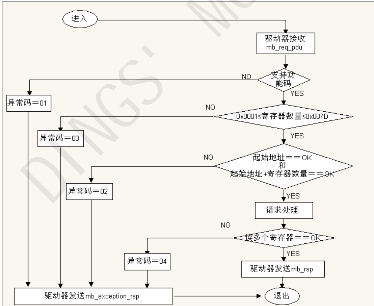
读保持寄存器的状态图
