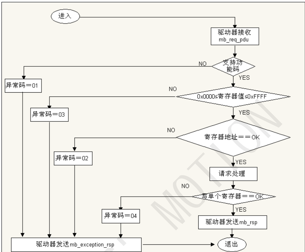
写单个寄存器状态图
