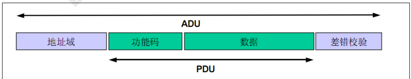
通用 MODBUS 帧
