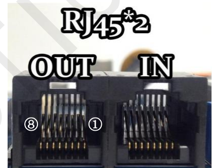
以面向插入视角看各针脚位置
