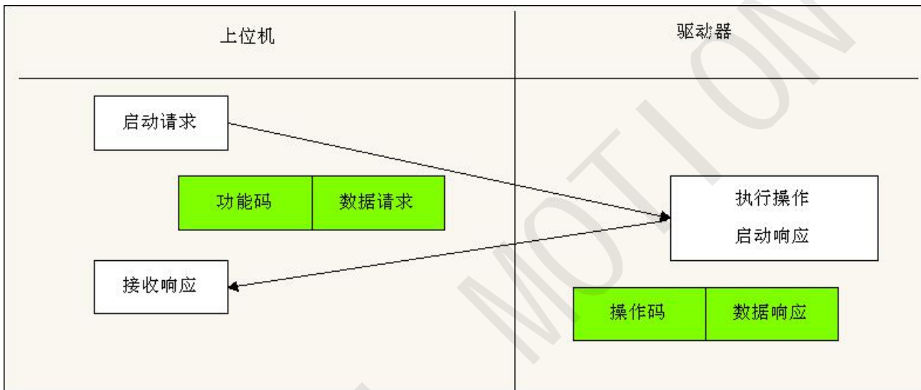
MODBUS 事务处理（无差错）
